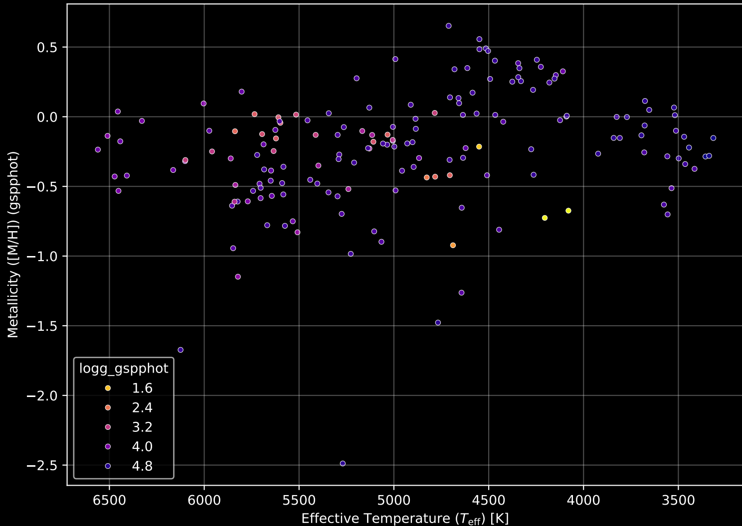
APOGEE DR17 Field: [SA57-S] Stellar Population Parameters (n= 169)
